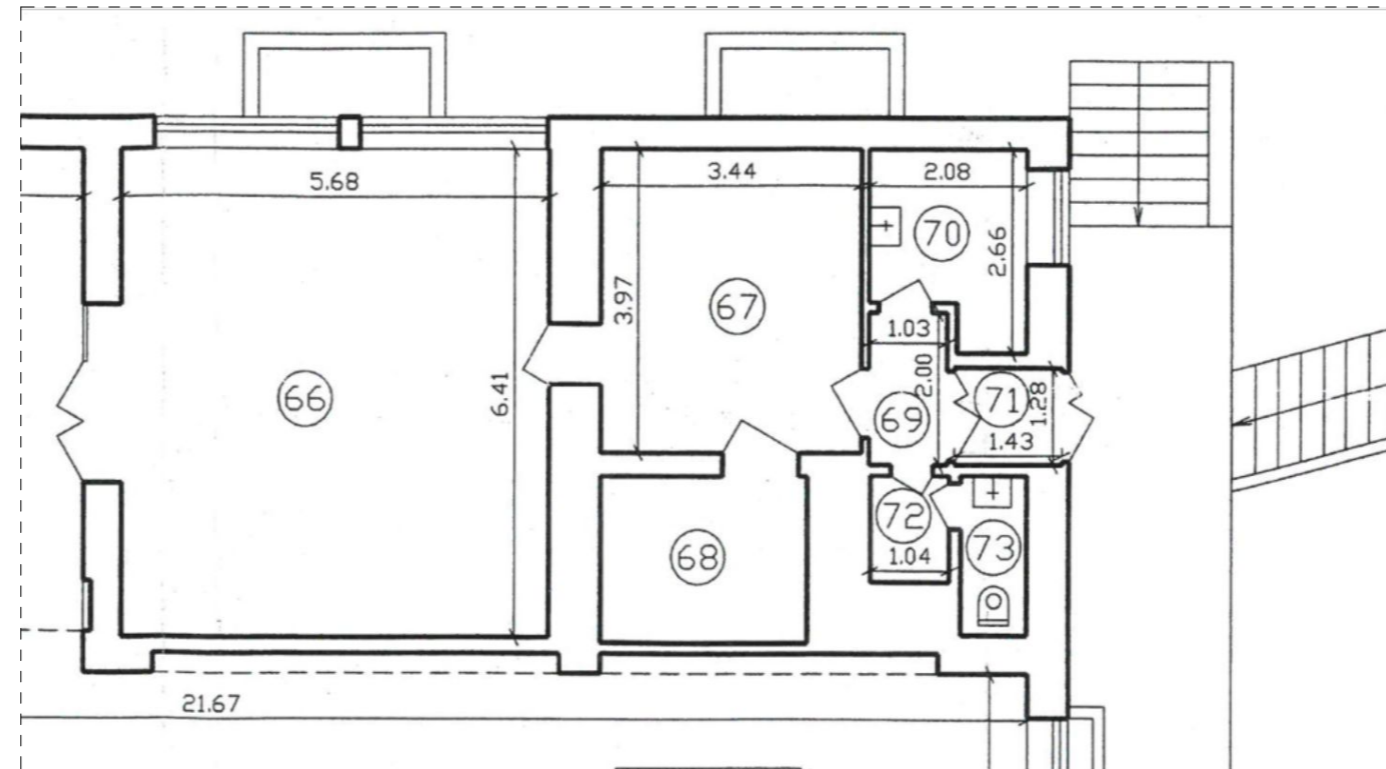
OLEMASOLEV OLUKORD M 1:100
